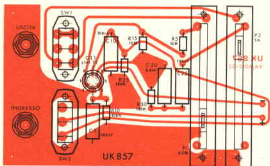
Fig. 2 - Serigrafia del circuito stampato.
