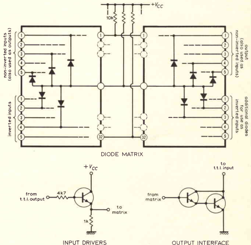
Fig. 12 - Schema elettrico semplificato del codificatore/decodificatore a matrice, in grado di convertire un segnale Murray in un segnale Elliott.
