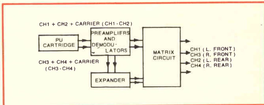
Fig. 10 - Sistema di decodifica a canali discreti del giradischi QZ 100 S.
