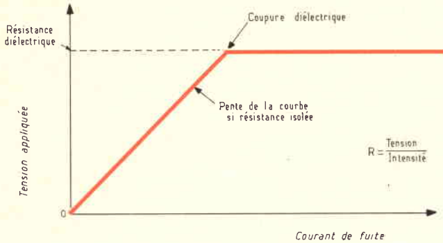
Fig. 9 - Il grafico mette in evidenza il fatto che la resistenza di isolamento e la rigidità dielettrica di un interruttore sono valori ben distinti fra loro.
