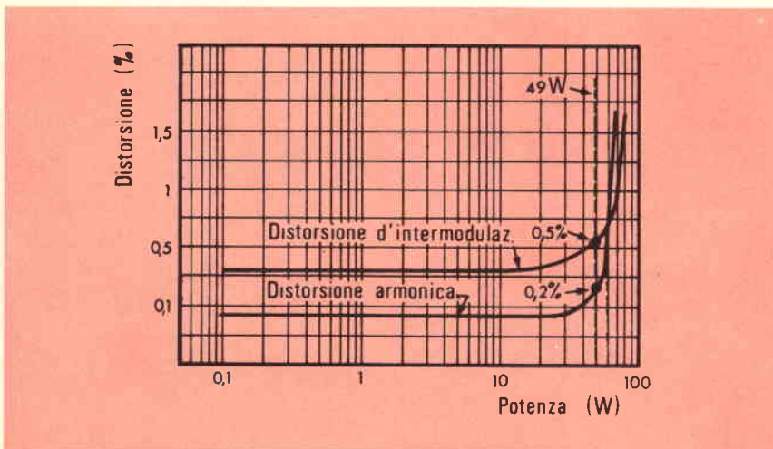
Curva della percentuale di distorsione armonica e d'intermodulazione
