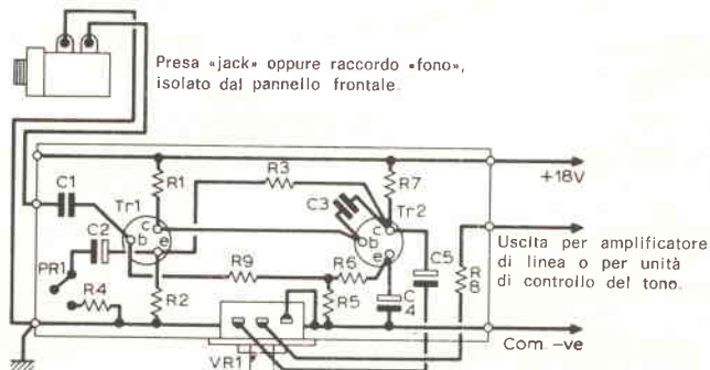
Fig. 18 - Bassetta a circuiti stampati, recante però questa volta i componenti che costituiscono la sezione di preamplificazione per testina magnetica di cui alla figura 17.
