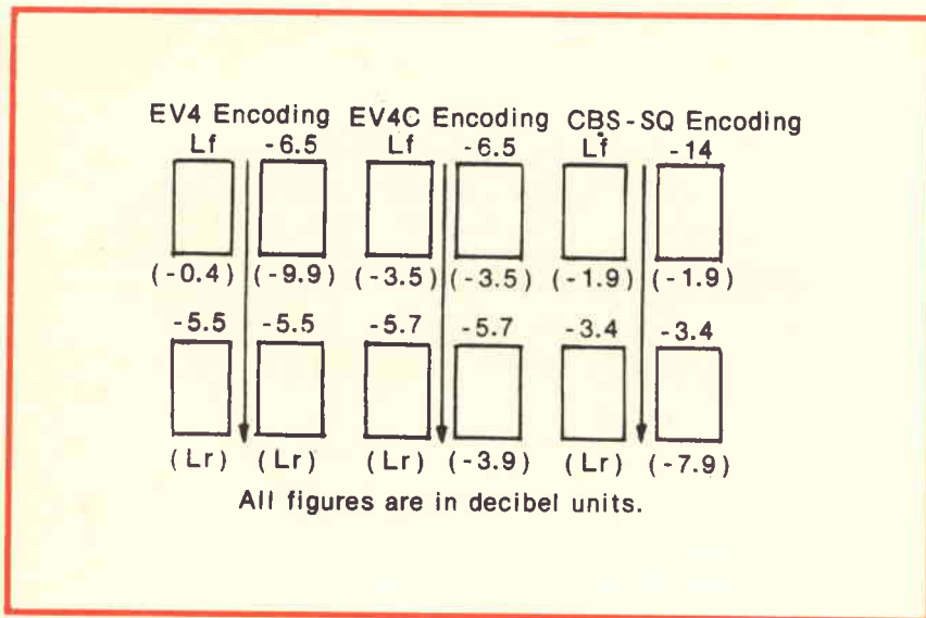
Fig. 11 - Sistema di decodifica a matrice del giradischi QZ 100 S.
