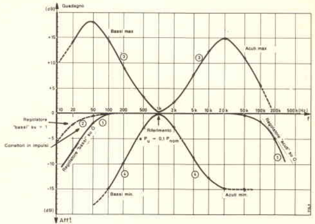
Fig. 3 - Banda passante BF e azione dei regolatori di toni.
