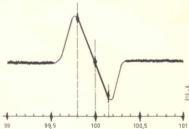
Fig. 6 - Risposta del discriminatore per un collegamento di 100 \mu V.
