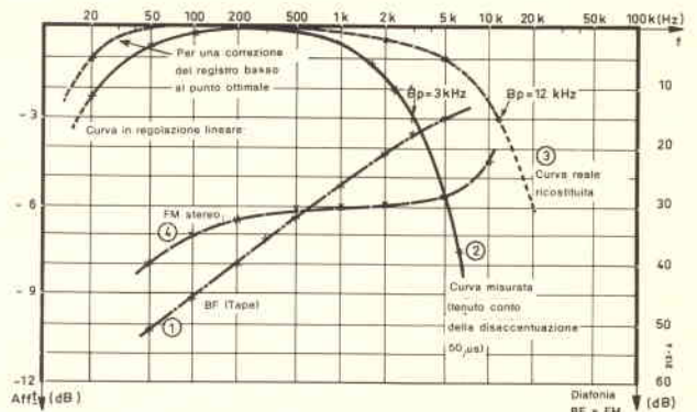
Fig. 4 - Banda passante globale, con e senza disaccentuazione, e curve di diafonia FM e BF.
