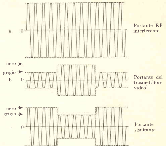
Fig. 4 - Spiegazione del fenomeno che dà luogo alla inversione dell'immagine (immagine negativa) in presenza di una forte interferenza.
