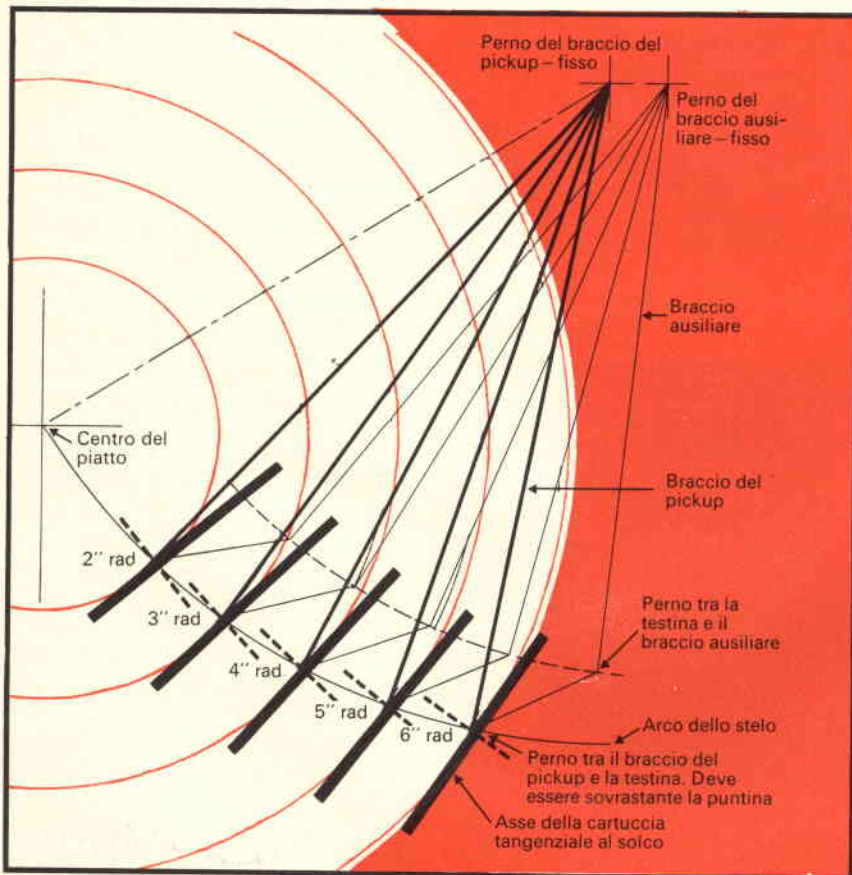
Fig. 4 - Geometria del «tracking» esattamente tangenziale del braccio dei giradischi della serie Zero 100.
