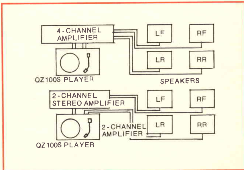
Fig. 9 - Collegamenti di un amplificatore quadrifonico o di due amplificatori stereo al giradischi QZ 100 S per ottenere un impianto quadrifonico.
