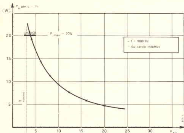
Fig. 1 - Curva di potenza media con segnale sinusoidale in funzione del carico.
