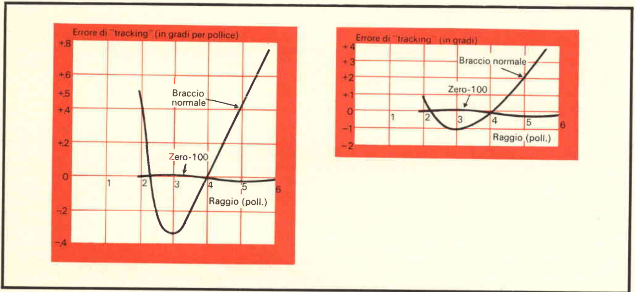
Fig. 3 - Confronto fra i diagrammi di «tracking» dei modelli Zero 100 e quelli di un braccio standard.
