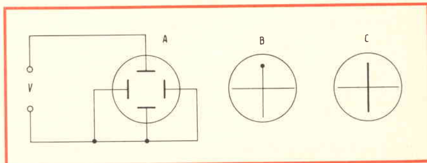
Fig. 1 - Collegamento di principio per effettuare misure di tensione mediante l'uso dell'oscillografico. B = punto caratteristico delle misure di una tensione continua. C = traccia caratteristica della misura di una tensione alternata.
