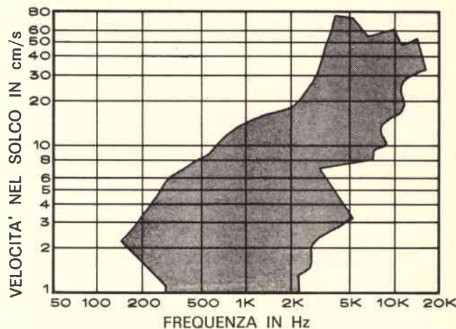
Fig. 4 - La zona tratteggiata visibile in questo grafico mette in evidenza i limiti della gamma di frequenza e di velocità che vengono riscontrati in un certo numero di dischi di produzione commerciale, che presentano elevate difficoltà agli effetti della «trackability». I tecnici della Shure Brothers' hanno eseguito queste misure per determinare l'attitudine da parte della testina a seguire il solco, per ottenere una buona riproduzione.
