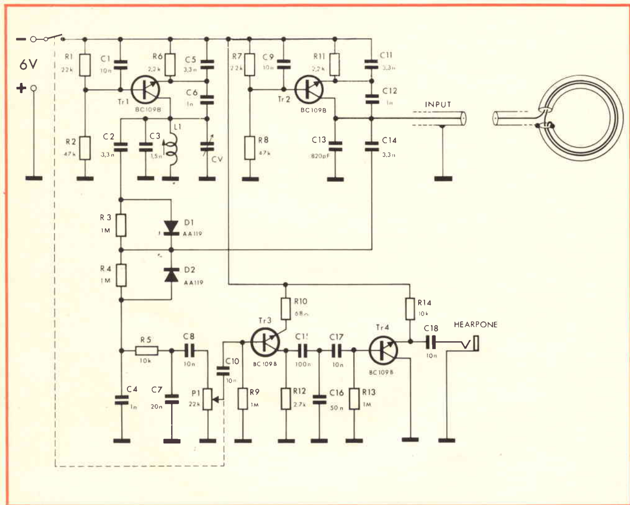
Fig. 2 - Schema elettrico del cercametalli AMTRON UK 780 reperibile presso tutti i punti di vendita dell'organizzazione GBC Italiana.
