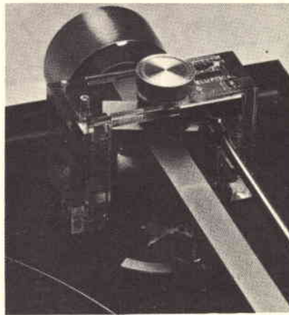
Fig. 2 - Sistema di compensazione magnetica antiskating, regolazione della forza d'appoggio della puntina sul disco e dispositivo ARC dei nuovi modelli della serie Zero 100.
