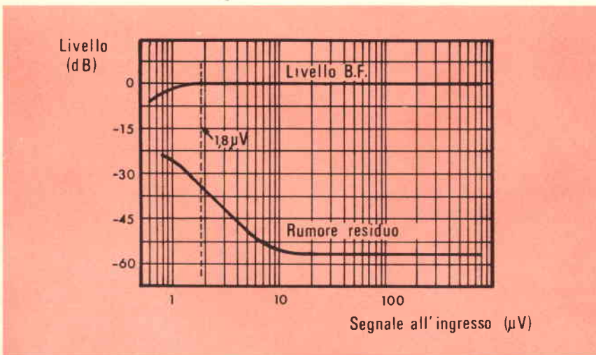
Curve di livello d'uscita BF e di rumore di fondo residuo della sezione FM, in funzione del segnale.
