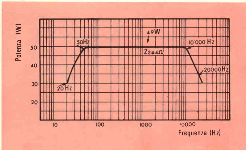
Curva di responso potenza/frequenza.
