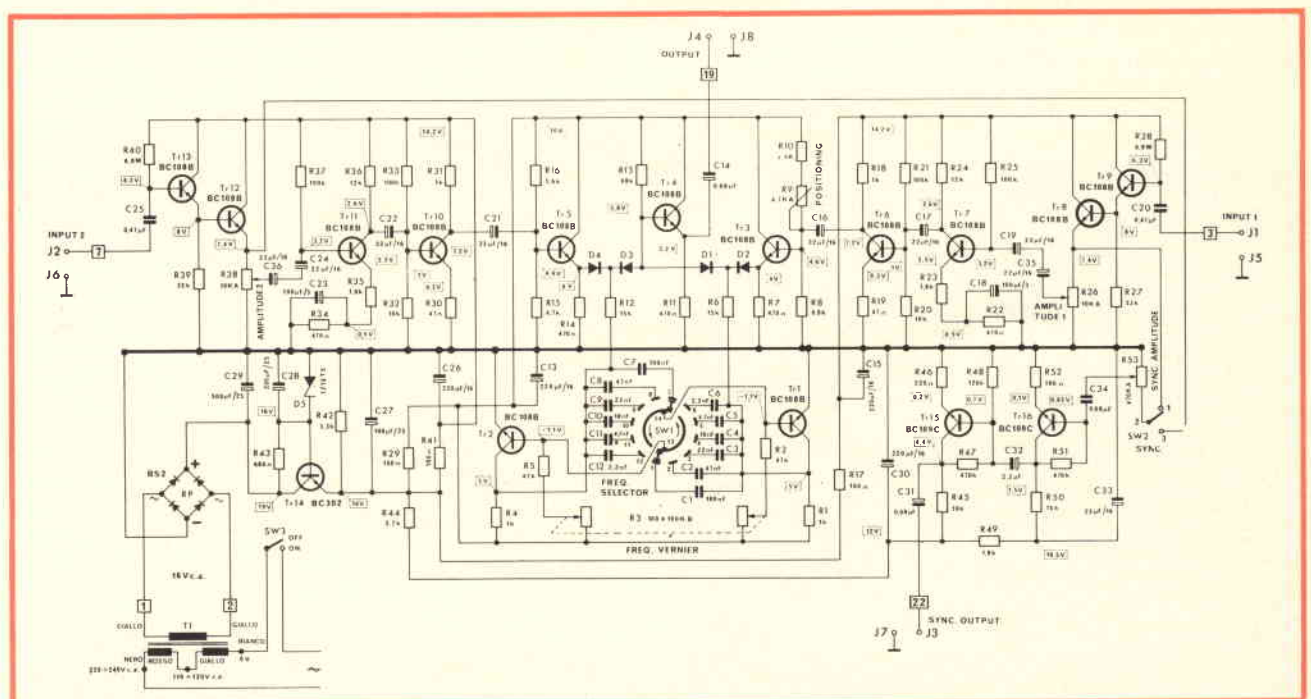
Fig. 1 - Circuito elettrico del commutatore AMTRON UK 585 (GBC Italiana) il quale permette di trasformare un oscilloscopio ad una traccia in un moderno oscilloscopio a due tracce.
