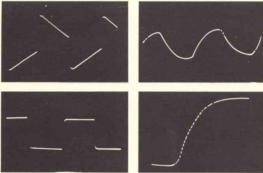
Fig. 1 - Comportamento, in regime rettangolare del sinto-amplificatore Elac 1000 TE. Dall'alto in basso e da sinistra a destra, segnali osservati a 40 Hz, 1.000 Hz, 10.000 Hz e 20.000 Hz; a 10.000 Hz i tempi di commutazione superano i 20 \mu s.
