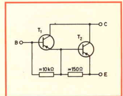
Fig. 5 - Schema elettrico caratteristico di un transistore Darlington integrato.
