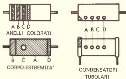
Fig. 10 - Sono rappresentati quattro diversi tipi di resistenze ad impasto, con identificazione dei metodi corrispondenti con i quali il valore intrinseco viene espresso mediante il codice a colori precisato nella tabella.
