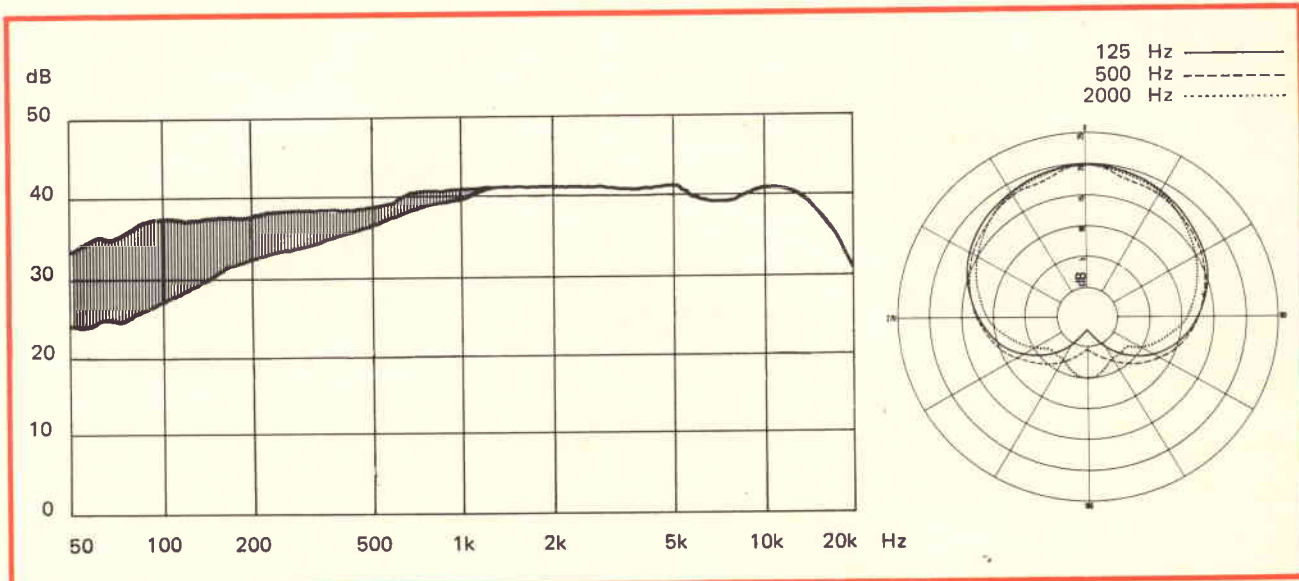
Fig. 9 - Curva di risposta secondo un diagramma polare nel piano orizzontale e di frequenza del microfono Revox 3400. Si noti la possibilità di taglio delle note basse introdotta dall'attenuatore accoppiato al microfono. La risposta di frequenza è contenuta entro \pm 3 dB da 30 a 17.000 Hz ed il diagramma polare è di tipo «cardioidide» con spiccati dati direzionali.
