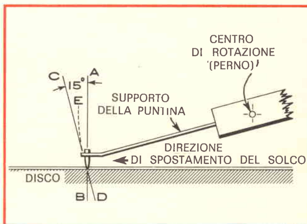
Fig. 5 - L'angolo verticale del «trancing» permette di descrivere il movimento di una puntina costretta a seguire le modulazioni verticali del solco. La linea a 15°, C-D, rappresenta il valore attualmente standardizzato dell'angolo di taglio per la registrazione dei dischi commerciali; la linea tratteggiata E-D viene prestabilita in funzione della posizione del perno intorno al quale ruota la puntina.
