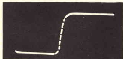
Responso ai segnali quadrati. Dall'alto in basso, a 40 Hz, 1000 Hz e 20.000 Hz; a 10 kHz il tempo di commutazione è di 5 µs.
