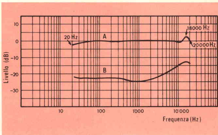
Curve di responso (A) e diafonia (B) della testina fonorivelatrice DM 101 MG.
