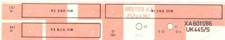
Fig. 3 - Serigrafia del circuito stampato CS2.
