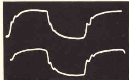
Questi oscillogrammi mettono in evidenza l'ottimo comportamento della testina fonorivelatrice Shure DM 101 MG.
