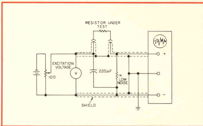
Fig. 7 - Caratteristiche di semplicità del circuito che soddisfa le esigenze della prova sistematica denominata «tap-testing». Per la realizzazione di questo circuito è naturalmente necessario usare componenti a bassa rumorosità intrinseca.
