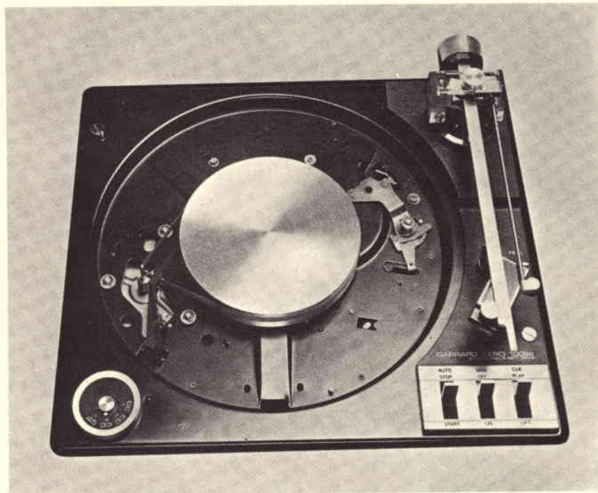
Fig. 6 - Sistema di trasmissione a cinghia per il giradischi Zero 100 SB.
