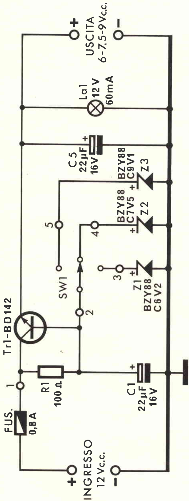
Fig. 1 - Schema elettrico.
