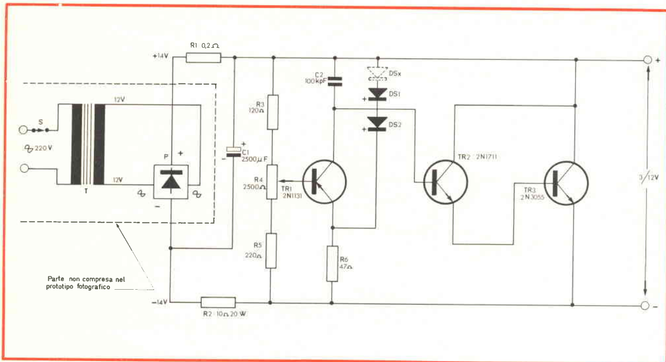
Fig. 2 - Schema elettrico.
