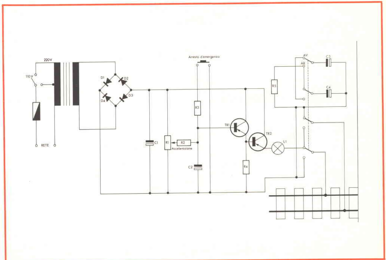
Fig. 2 - Schema elettrico di un altro circuito di regolazione della velocità dei trenini elettrici.
