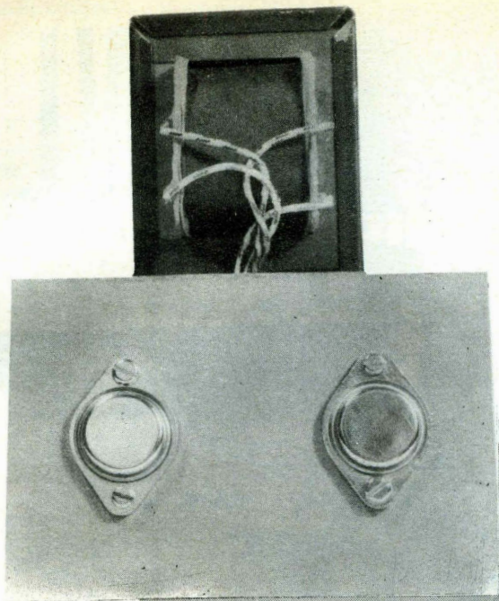
A lato: chassis dell'alimentatore: si scorgono i due transistor di potenza bloccati sul lato posteriore della scatola che funge oltre che da supporto, anche da radiatore.
