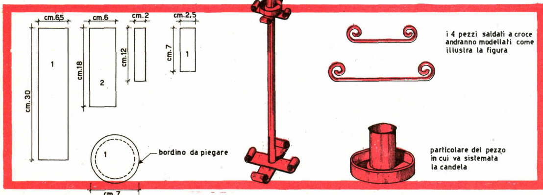
forma da dare alla striscietta cm.14x1,5
