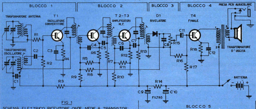
SCHEMA ELETTTRICO RICEVITORE ONDE MEDIE A TRANSISTOR
