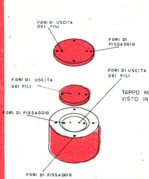
5 - Un conveniente tipo di scatola di accensione.
