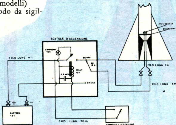
1 - Un funzionale sistema di accensione del razzo.
