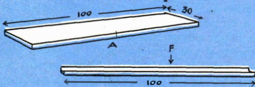
Fig. 7. Elementi formanti il supporto per la vasca: a) piano di base; b,c) sostegni laterali; d) cornici semicircolari; e) alloggiamento per i cuscinetti a sfere; (diam. 42 mm.) f) strisce di rinforzo.
