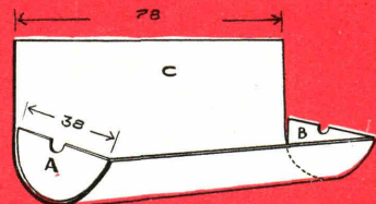
Fig. 5. Elementi costituenti la vasca semicilindrica in plexiglass: a,b) semicerchi; c) foglio da fissare ai semicerchi mediante l'apposito mastice.
