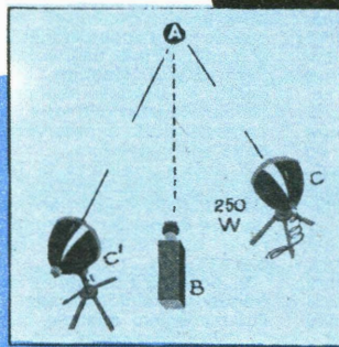
Ripresa in interni con l'uso di due lampade. A) soggetto, B) cinepresa, C, C') lampade stasate
