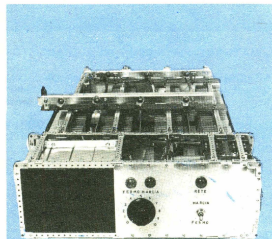
Fig. 1 - Veduta del pannello frontale e d'insieme dell'azionamento da 20 kw. AZ-01/18. Le scatole a sinistra contengono il circuito elettronico.
