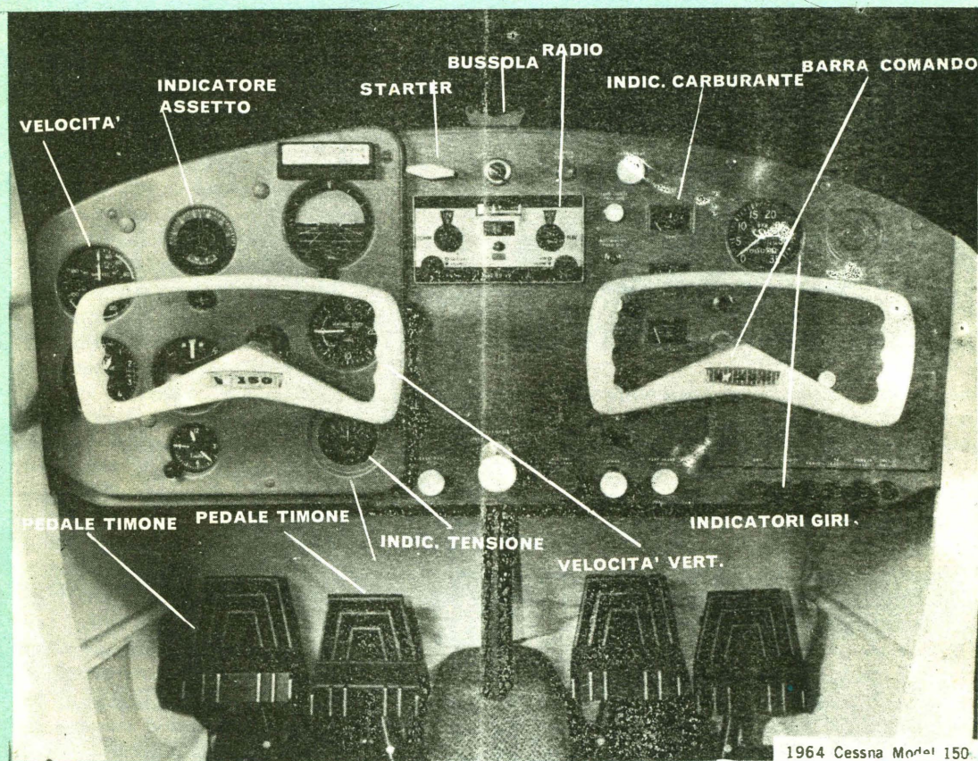
Fig. 6 - Vista del pannello di comando di un aereo da turismo a doppia guida; nella foto sono indicati i comandi principali. L'aereo è un Cessna 150.
