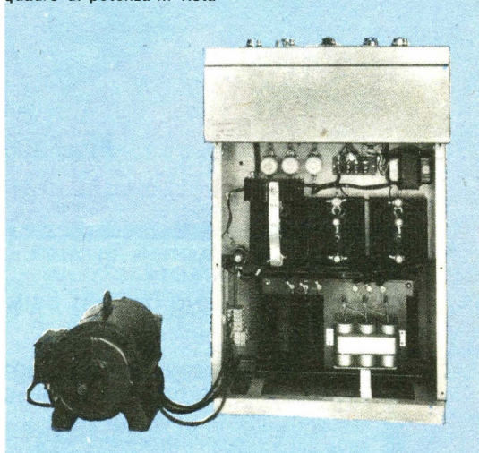
Fig. 2 - Azionamento AZ-01/5: Veduta d'insieme con quadro di potenza in vista
