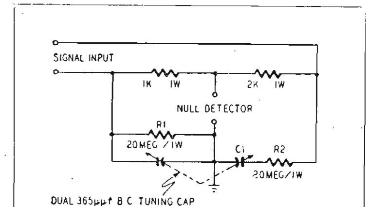
Circuito del ponte di Wien modificato descritto, nel quale in luogo di un tandem di resistenze variabili è adoperato un condensatore variabile doppio e le normali posizioni di C1 e C2 risultano invertite.
