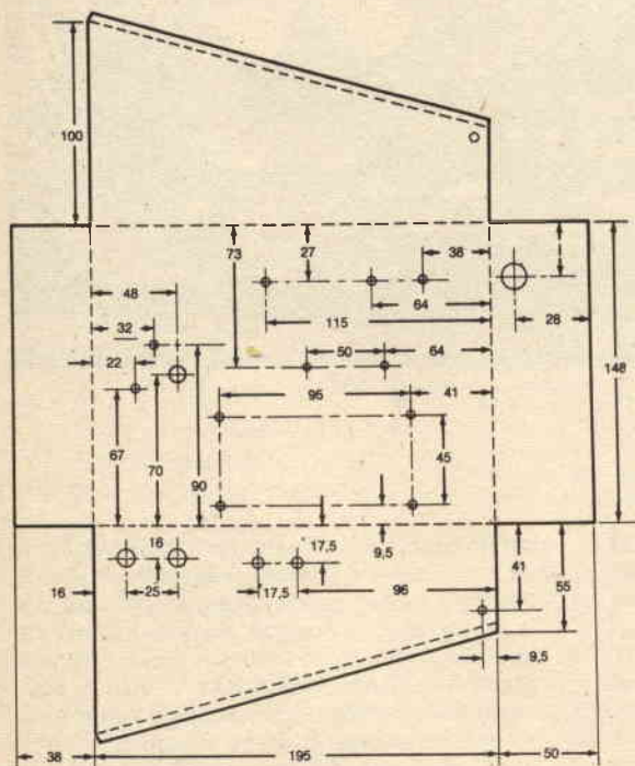
Fig. 4 - Particolari costruttivi del telaio.
