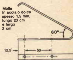
Fig. 5 - Particolari costrutti del pedale di legno e della molla. I due fori praticati nel pedale servono per il fissaggio della maschera. La molla serve a far ritornare in alto il pedale quando il piede viene sollevato.
