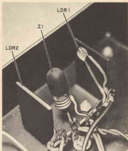
La lampada I1 è verniciata di nero opaco. Per illuminare i fotoresistori, si asportano puntini di vernice ai lati della lampada. I punti in cui la vernice è stata asportata, in questa fotografia appaiono neri.
