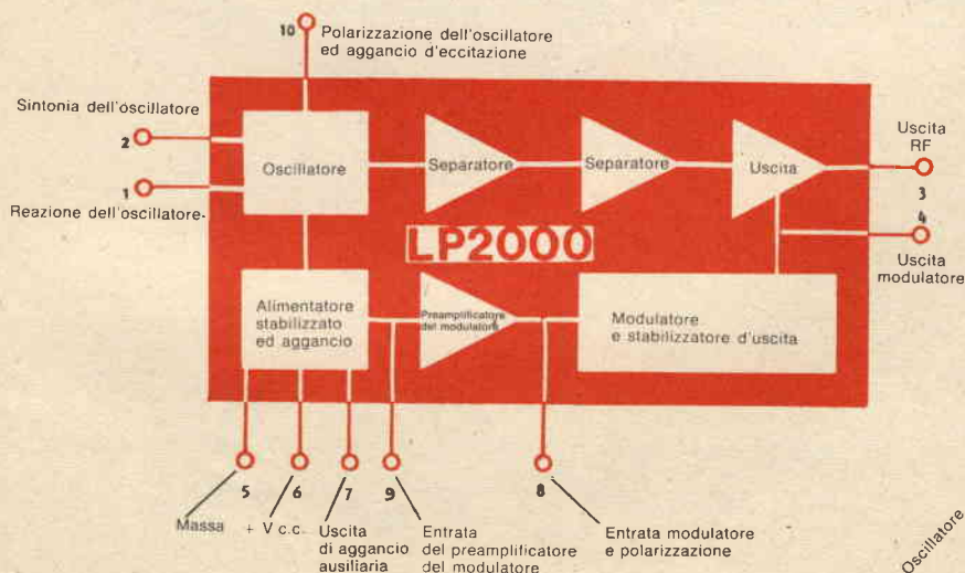
Fig. 1 - Schema funzionale a blocchi del microtrasmettitore LP2000 della Lithic.
