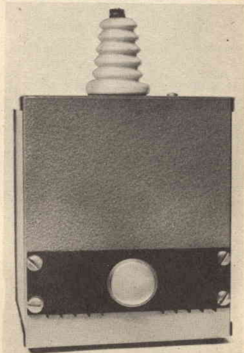
Fig. 5 - Il transistor è elettricamente isolato dal radiatore di calore e questo è fissato alla parte posteriore della scatola. L'involucro (collettore) di Q1 non deve entrare in contatto con parti metalliche.
