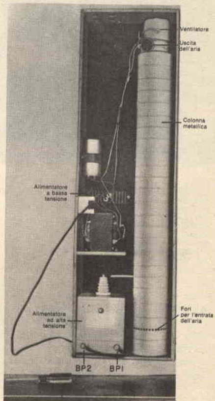
Fig. 7 - Per ragioni estetiche, i barattoli di caffè sovrapposti sono stati verniciati prima di montarli nel mobiletto. I quattro fori di ventilazione nel pannello superiore servono per il raffreddamento dell'alimentatore.
