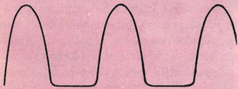
Distorsione inserita - Controllo R6 al minimo - Entrata 30 mV
