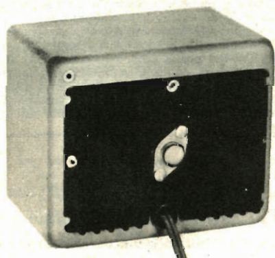
Per una buona dissipazione del calore, Q3 si monta su un radiatore di calore il quale funge anche da pannello posteriore della scatola.
