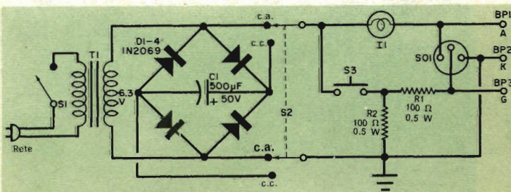
Fig. 1 - In questo strumento per la prova dei raddrizzatori controllati al silicio (SCR), progettato da un nostro lettore, vengono usati alimentatori sia c.a. sia c.c.
