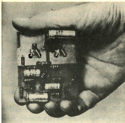
Questo piccolo amplificatore, nel quale viene utilizzato il nuovo economico transistor Texas Instruments, può fornire 2 W se si usa il circuito stampato come radiatore di calore.
