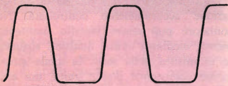
Distorsione inserita - Controllo R6 al minimo - Entrata 60 mV
