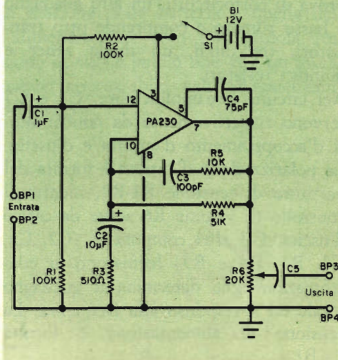
Fig. 3 - In questo circuito amplificatore, descritto in un bollettino tecnico della General Electric, viene usato un circuito integrato PA230. Si tratta di un amplificatore audio a basso livello, d'uso generale, con guadagno pari a 100.
