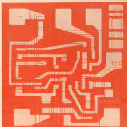
Il comparatore differenziale duale \mu\text{A} 711 della SGS, riprodotto nella fotografia, ha un ingresso comune e due ingressi indipendenti.
