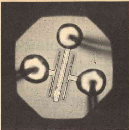
Fig. 4 - Ecco la caratteristica configurazione del transistore MOS FET ad effetto di campo FI100.
