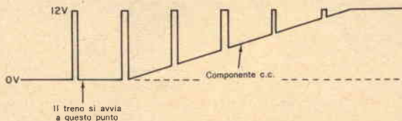
Fig. 2 - Il gruppo che presentiamo produce un treno di impulsi stretti, in aggiunta alla potenza c.c. variabile. Gli impulsi sono chiaramente visibili quando il regolatore è chiuso, ma scompaiono gradatamente quando il regolatore è al massimo. L'aumento istantaneo dell'impulso da zero al massimo garantisce una potenza immediata di valore tale da far funzionare il treno quando la manopola di scorrimento è aperta.
