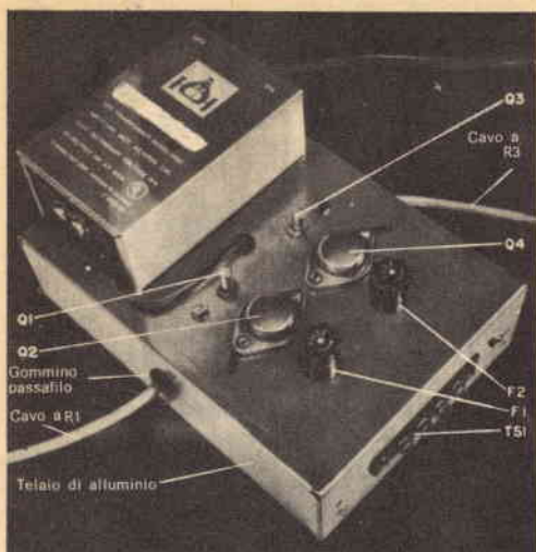
Fig. 2 - Sul telaio vi è spazio sufficiente per il gruppo trasformatore raddrizzatore. Montate Q2 e Q4 su radiatori di calore e Q1 e Q3 su zoccoli. I cavi che fuoriescono dai lati del telaio vanno ai dispositivi di controllo della velocità.
