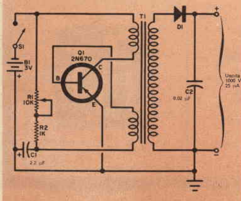
Fig. 1 - Semplice circuito convertitore c.c. - c.c. che eleva a 1.000 V la tensione della batteria.
