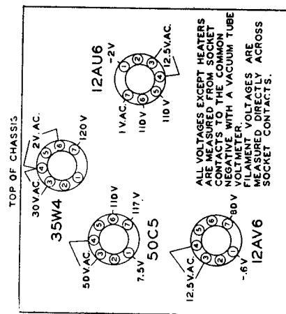
VOLTAGE TABLE
