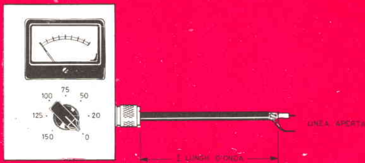
Fig. 5 - Per trovare una lunghezza di 1/4 d'onda l'estremità del cavo non deve essere cortocircuitata e lo spezzone sarà esattamente lungo 1/4 d'onda quando con il potenziometro sullo ZERO la lancetta non indicherà nessun passaggio di corrente.
