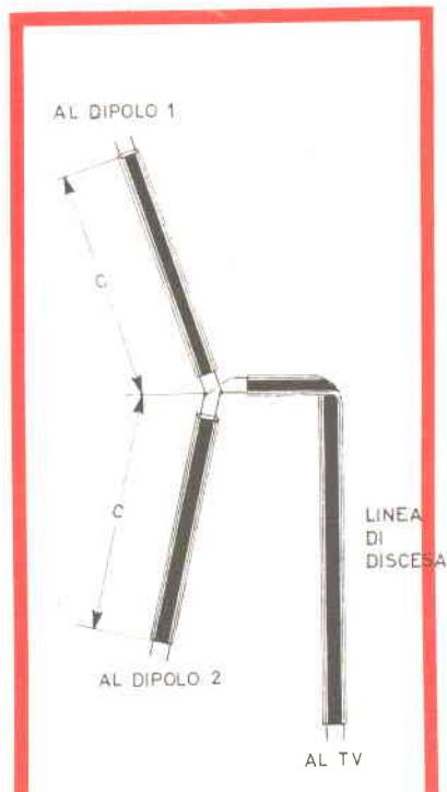
Fig. 3 - Le due antenne, siano esse sovrapposte o affiancate, dovranno essere collegate alla linea di discesa per mezzo di due spezzoni di piattina di uguale lunghezza. Anche la loro misura è critica ed è proporzionale alla lunghezza d'onda che si deve ricevere. In pratica ogni spezzone potrà essere lungo indifferentemente 1,26 - 2,10 - 2,94 - 3,78 volte la lunghezza del dipolo di cui sono dotate le antenne stesse.
