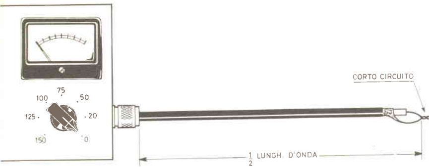
Fig. 3 - Lo spezzone di cavo sarà esattamente lungo una mezza onda quando con il potenziometro regolato sullo ZERO lo strumento non segnerà corrente.
