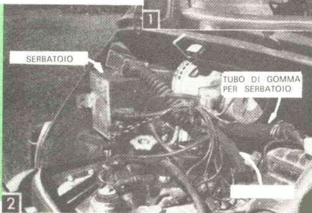
Figg. 1-2 - Nelle due foto è visibile il serbatoio supplementare che ci ha permesso di migliorare il sistema di raffreddamento di una 600, tanto da poter sopportare i lunghi percorsi dell'« Autostrada del Sole ».
