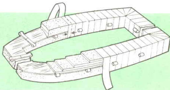
Fig. 2 - Applicate sopra e sotto al telaio dei pezzi di poliestirolo espanso incollandoli con vinavil.
