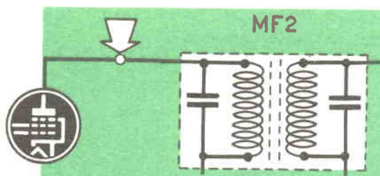
Fig. 3 - In un ricevitore a valvole, il nostro soppressore di disturbi può essere collegato direttamente sulla placca dell'ultima amplificatrice di MF e la massa.
