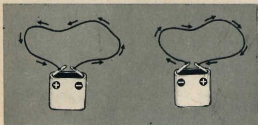
Fig. 9 - Nei conduttori metallici, contrariamente a quanto avviene nelle valvole, gli elettroni possono fluire in entrambi i versi. Infatti, in qualunque modo si inserisca la pila ai capi di un conduttore metallico, la corrente fluisce ugualmente in ogni caso attraverso il conduttore.
