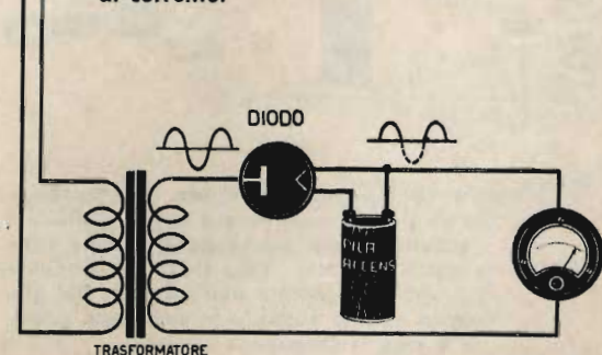
Fig. 11 - Con il diodo è possibile trasformare una corrente alternata in una corrente unidirezionale intermittente. In questo caso il diodo funziona da valvola raddrizzatrice di corrente.
