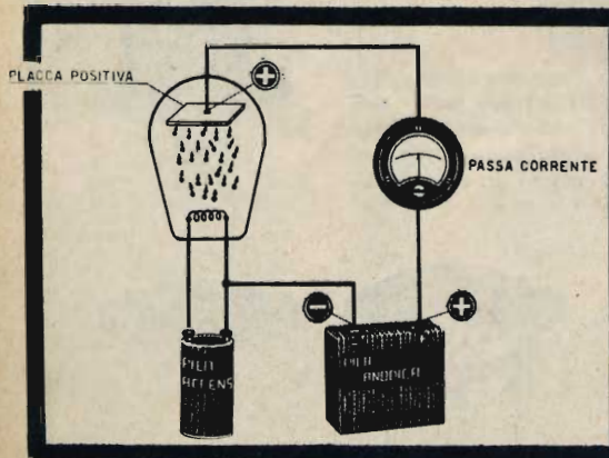
Fig. 7 - Il fenomeno del flusso elettronico nell'interno della valvola si verifica solo se alla placca è applicata una tensione positiva. In questo modo gli elettrodi, emessi dal filamento, possono essere attratti dalla placca e formare una corrente tra il filamento e la placca.
