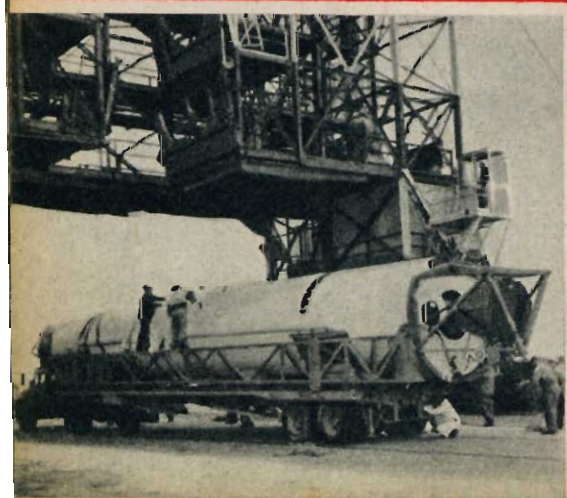
Sopra: Per salire e scendere dal « ventre » dell'aereo, il missile vien fatto scorrere su di un carrello guidato da una rotaia. Sotto: Dopo 20 ore di volo, il Thor ha finalmente raggiunto la torre della sua base di lancio.
