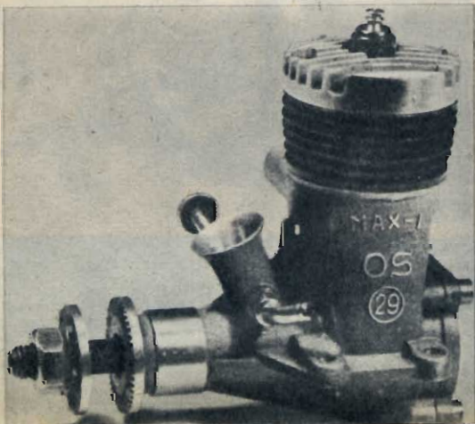
Fig. 13 - Il G32 da 1 cc. di produzione italiana. Motore dalle eccezionali caratteristiche, popolarissimo fra gli aeromodellisti italiani per il basso prezzo (L. 4500), il basso consumo e l'alto rendimento. 0,10 HP di potenza.
