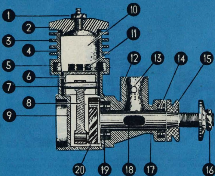
Fig. 5 - La sezione di cui a figura ci fornisce — in rapida analisi — idea delle parti costituenti il motore: 1. Candela; 2. Testa del motore; 3. Alette di raffreddamento; 4. Camicia; 5. Luci di scarico; 6. Pistone; 7. Splnnotto; 8. Biella; 9. Carter; 10. Camera di scoppio; 11. Luci di travaso; 12. Carburatore; 13. Venturi del carburatore; 14. Cuscinetto a sfere anteriore; 15. Supporto godronato; 16. Dado ferma-elica; 17. Bronzina; 18. Valvola rotativa; 19. Cuscinetto a sfere posteriore; 20. Albero manovella.
