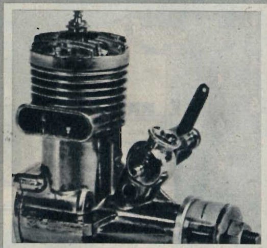
Fig. 3-4 - Motori per aereomodellismo con incorporato il dispositivo di regolazione della velocità di rotazione del Pelica. Tale dispositivo viene soprattutto utilizzato nel caso in cui si abbiano a disposizione modelli radiocomandati.
