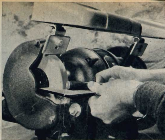
Se siete un artigiano vi conviene avere una mola da banco. Essa deve avere l'attrezzatura qui illustrata: una copertura che circonda le ruote e schermi contro schegge di vetro e scintille.
