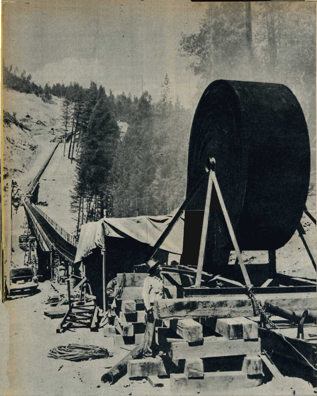
STRADA DI GOMMA Un nastro trasportatore di gomma, della lunghezza di 5.400 metri trasporterà 20 milioni di tonnellate di terra di riempimento ricavata dalle pendici d'una montagna fino a una diga che si sta costruendo in California. Nella fotografia: gli ingegneri incaricati del lavoro fanno svolgere da un rullo il nastro di gomma, largo 107 centimetri nella località detta Trinity River, nella quale ha inizio la discesa del nastro dalla vetta, per 2550 metri.
