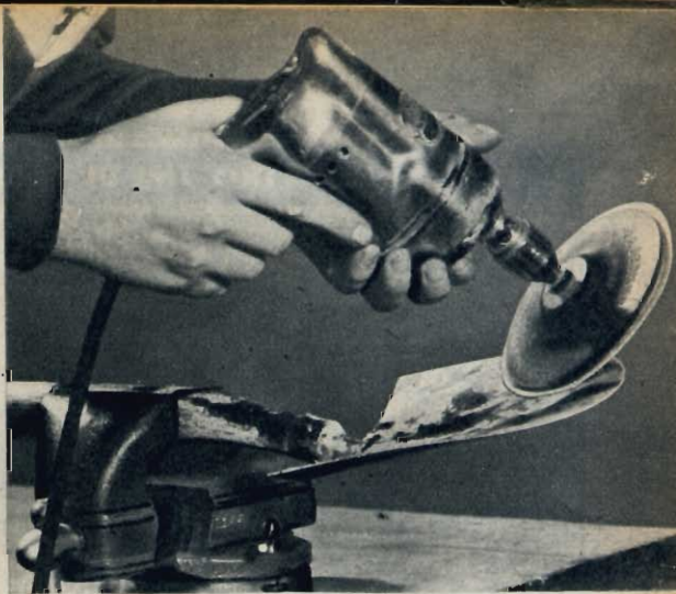
Un disco flessibile di smerigliatrice adattato ad un trapano elettrico può servire per affilare rapidamente utensili per giardinaggio. Non va usato in realtà come affilatore da taglio, ma soltanto per ripassare larghe superfici.
