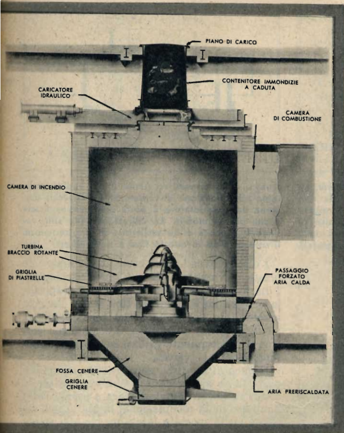
A sinistra: Veduta spaccata della camera di accensione nella quale le immondizie vengono distrutte e trasformate in gas combusti ed in cenere per quelle sostanze non combustibili. Sotto: Veduta esterna di uno stabilimento di incenerimento.
