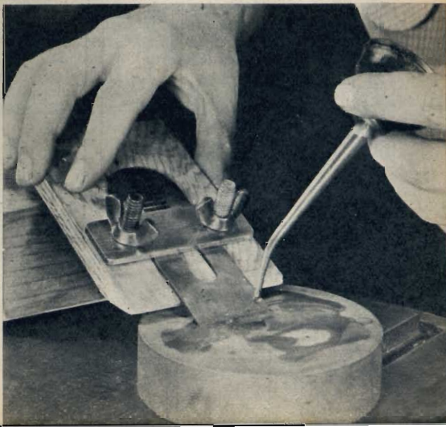
Questa piccola ruota di mola azionata da un motore veloce serve per affilare utensili di profilo irregolare. Serve anche per togliere le intaccature dall'orlo curvo di teste di fresa e simili.
