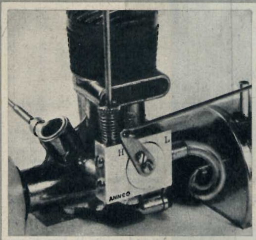
Fig. 3-4 - Motori per aereomodellismo con incorporato il dispositivo di regolazione della velocità di rotazione del Pelica. Tale dispositivo viene soprattutto utilizzato nel caso in cui si abbiano a disposizione modelli radiocomandati.
