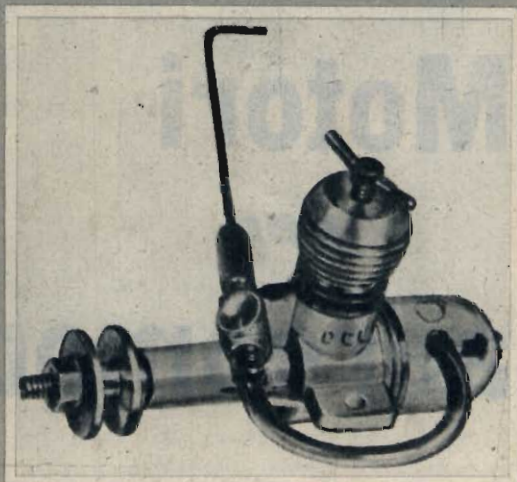
Fig. 1 - Motore ATWOOD, 0,8 cc., con serbatoio posteriore incorporato. Questo motore, che risulta senza dubbio uno dei migliori della sua specie, ha raggiunto grande popolarità in America. Il suo prezzo si mantiene inferiore alle duemila lire. — Fig. 2 - Il più piccolo motore del mondo: cilindrata 0,15 cc.
