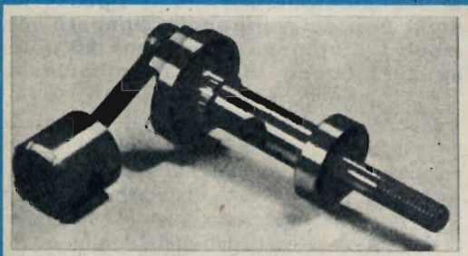
Fig. 9 - L'MC. COY con fasce elastiche, il che è deducibile dal reticolo che forma la camicia (visibile attraverso lo scarico) e che si rende necessario per la tenuta in sede dei segmenti (o fasce elastiche).
