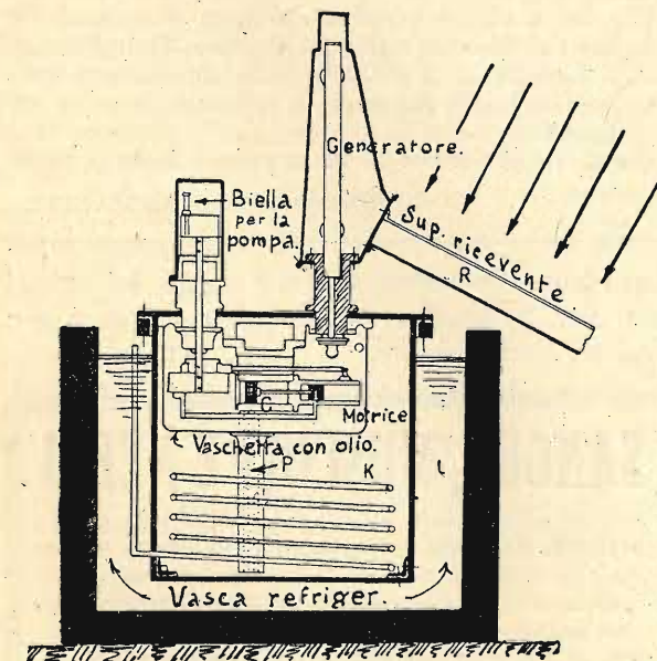
Fig. 1. — Schema dell'eliopompa.
