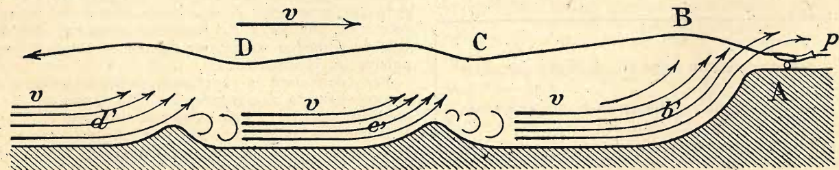
Fig. 37. — Traiettoria di un planeur contro un vento periodicamente ascendente.
