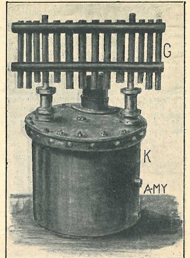
Fig. 2. — L'eliopompa senza radiatore.
