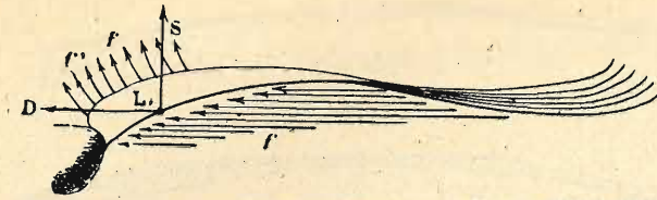
Fig. 11. — r , superficie laterale obliqua; f, f' , filetti fluidi; S , forza sollevatrice; D , componente di derivazione.
