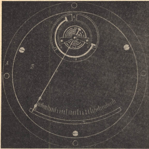
Fig. 1. — Parte anteriore dell'apparecchio (è visibile il sistema di smorzamento, la scala ed i due indici) prima della carcassa protettrice.
