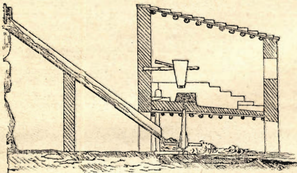
Fig. 1. — Motrice a ritrecine.
