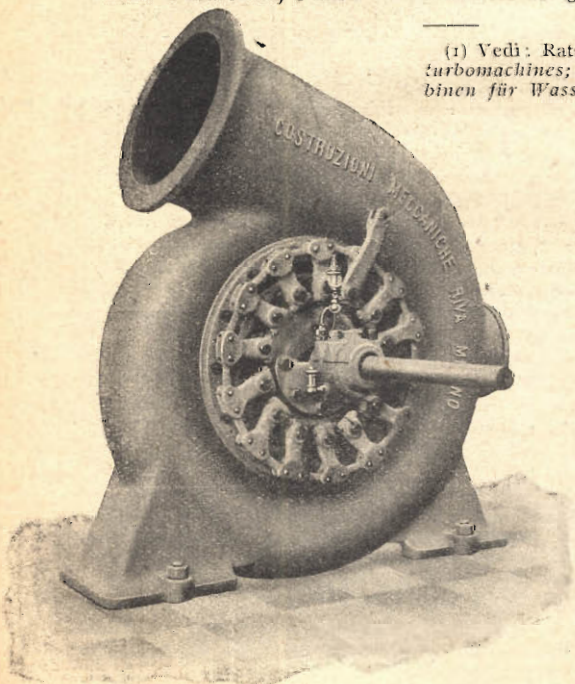
Fig. 11. — Turbina con distributore a comando esterno.
