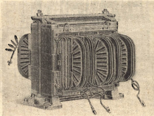
Fig. 5. — Trasformatore trifase con raffreddamento ad aria.
