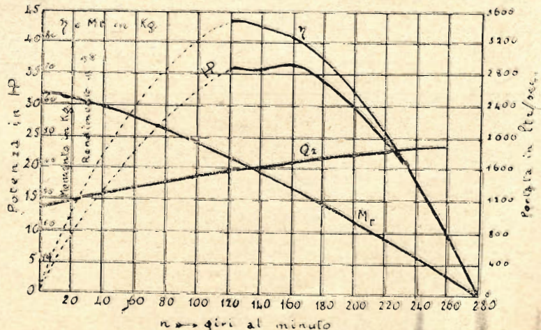
Fig. 3. — Curve caratteristiche di una turbina di Escher & Wyss. — H=2 m. D=500 mm.
