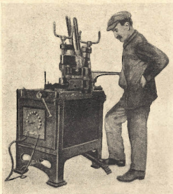
Fig. 1. — Macchina usuale.
