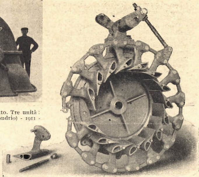
Fig. 12. — Distributore con comando a catena.
