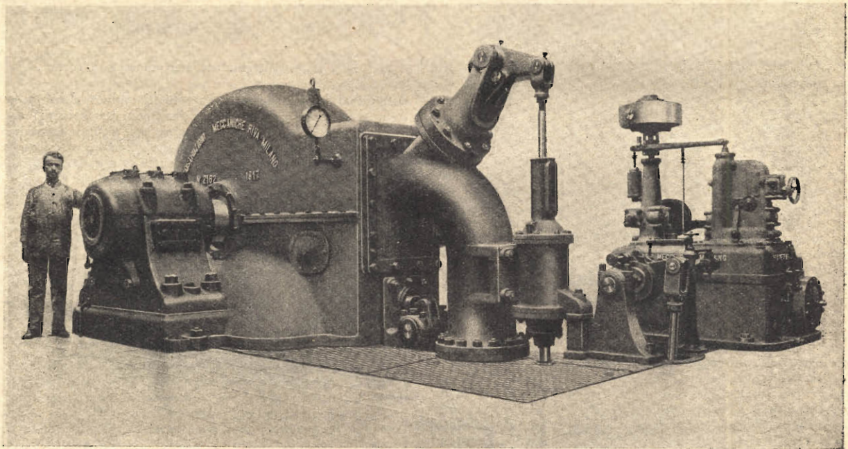
Fig. 14. — Turbina 14 000 HP - caduta m. 525 - per l'impianto Lys della Soc. Italiana Ernesto Breda.
