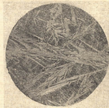
Martensite e austenite.
