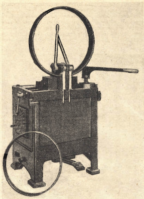
Fig. 4. — Macchina per cerchi d'automobile.
