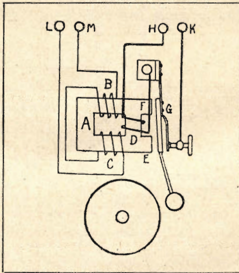
A , nucleo; B-C , avvolgimento primario; D , avvolgimento secondario; E-F , appendici polari; G , ancora; H-K , rete a bassa tensione; L-M , rete ad alta tensione.
