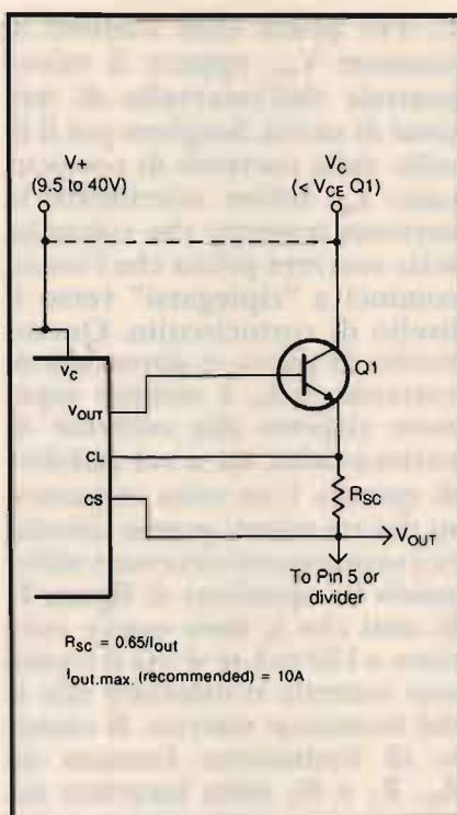
8 Un singolo transistor di potenza esterno collegato al 723.
