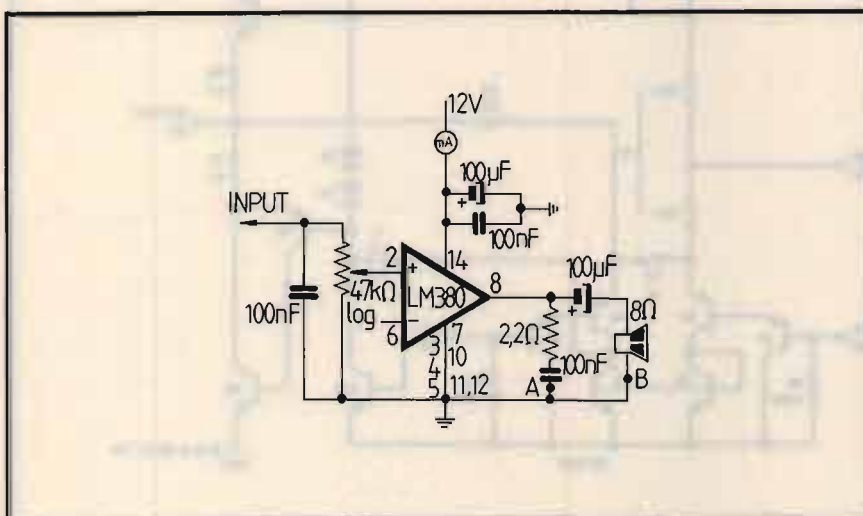
② Circuito amplificatore audio con LM380.
