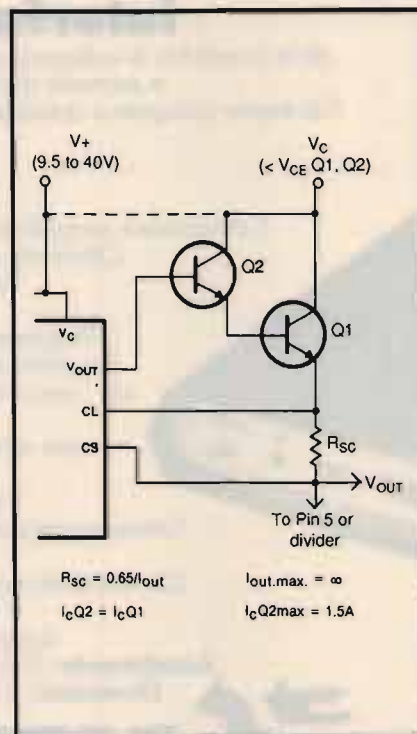
9 Una coppia di transistor fornisce migliori prestazioni rispetto al circuito di figura 8 ed è consigliabile per alimentatori con corrente massima erogata superiore a 5 A.
