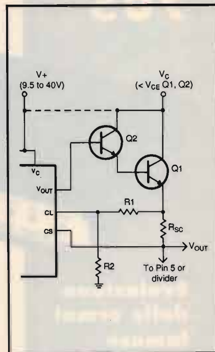
10 La limitazione di corrente a ripiegamento applicata a un circuito con transistor di potenza esterno.
