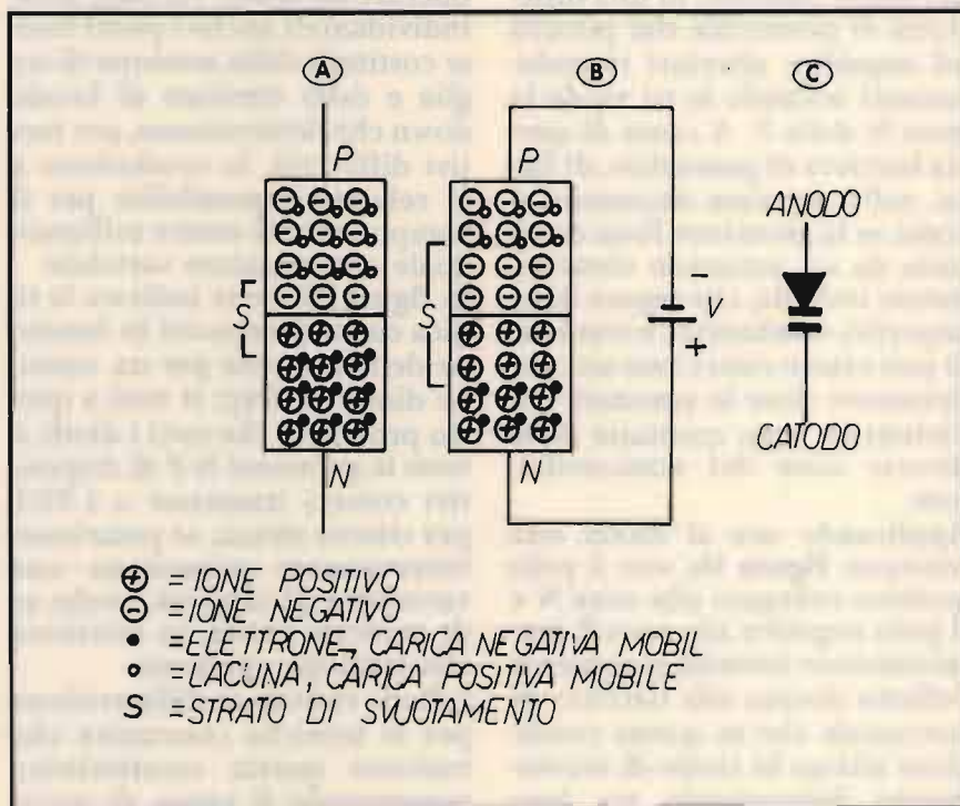
① a) struttura semplificata di un diodo non polarizzato con indicazione, non in scala, dello strato di svuotamento; b) il medesimo diodo a cui viene applicata una polarizzazione inversa per mezzo del generatore V, si noti l'estensione dello strato di svuotamento; c) simbolo grafico convenzionale del diodo Varicap.
