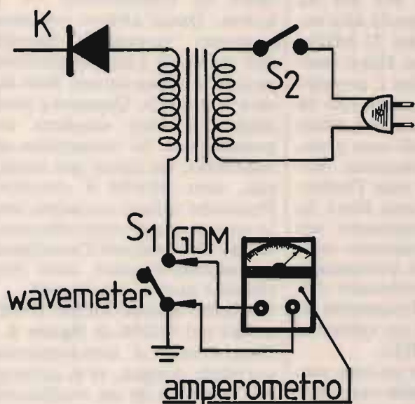
figura 2 Per controllare la corrente anodica si può collegare l'amperometro fra i contatti dell'interruttore S1, che serve a togliere la tensione sulla placca quando l'apparato funziona come ondometro. La corrente anodica deve aumentare se si toglie la bobina del circuito oscillante del GDM. Se la corrente non varia, l'oscillatore non funziona.
