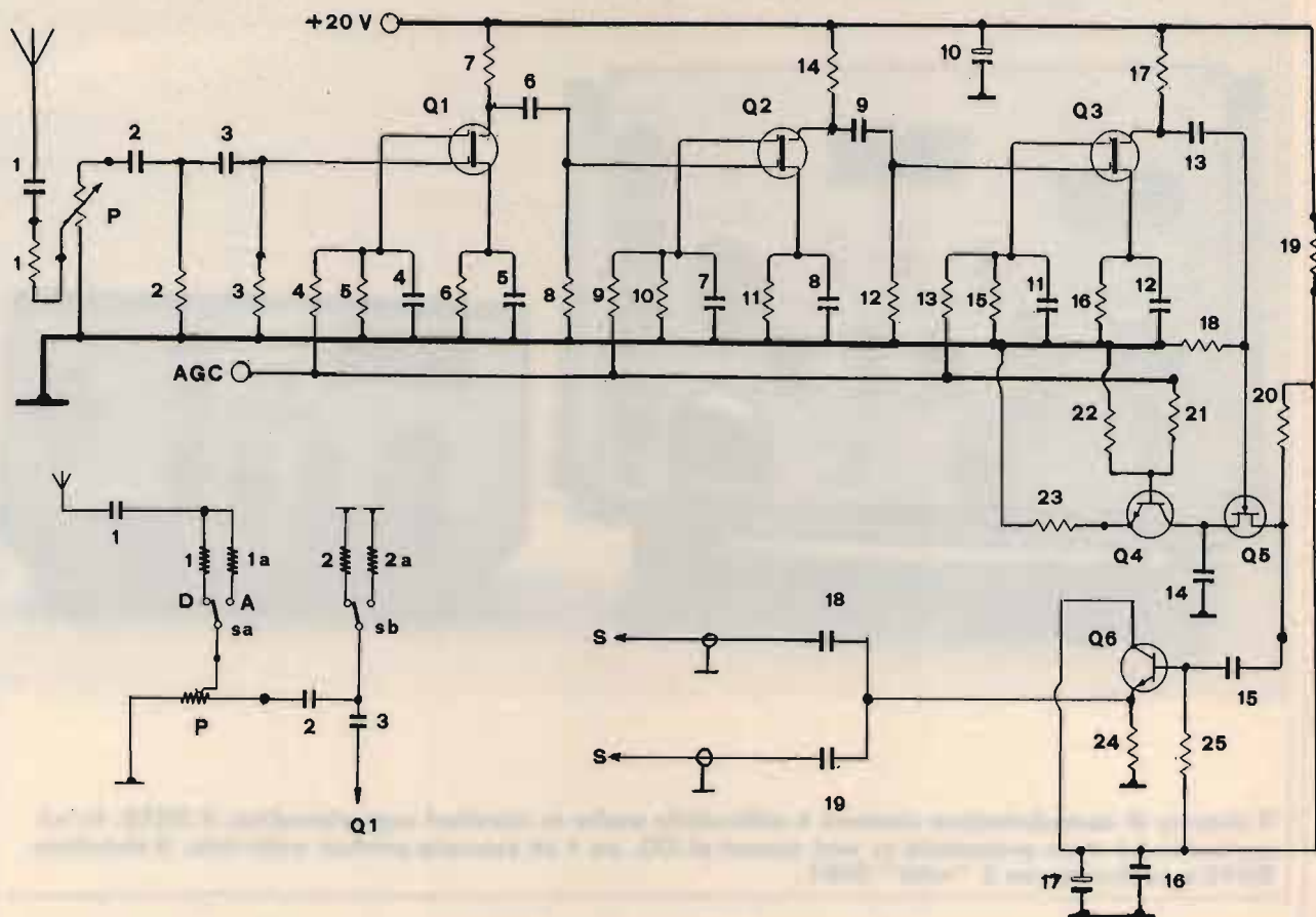
Schema elettrico dell'amplificatore di alta frequenza. In basso a sinistra, la variante dell'attenuatore di segnale in entrata.
