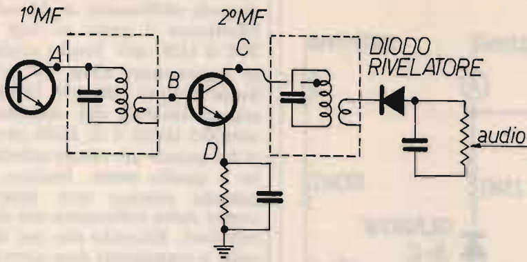
figura 3 Schema semplificato del primo e secondo stadio di media frequenza di un ricevitore per onde medie. Sul collettore del secondo transistor (C) il segnale è piuttosto forte e lo si può facilmente misurare con il probe. Il segnale può essere anche ascoltato con una cuffia collegata all'uscita del probe.
