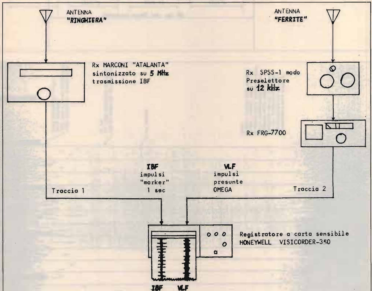
figura 7 Disposizione delle apparecchiature usate per ottenere il confronto degli impulsi delle presunte Stazioni Omega con gli impulsi "marker" di 1 sec, trasmessi da IBF (Torino). Vedi anche figure 8 e 9.
