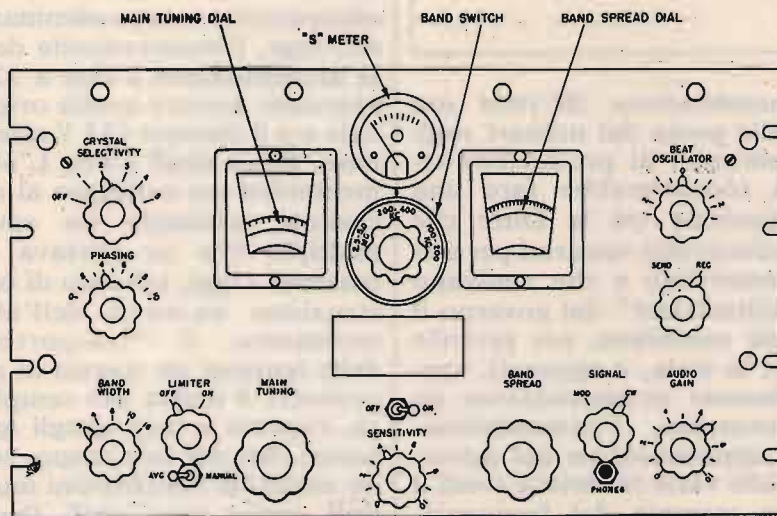
figura 1 Vista frontale del BC1004, e principali comandi e indicatori sul pannello.
