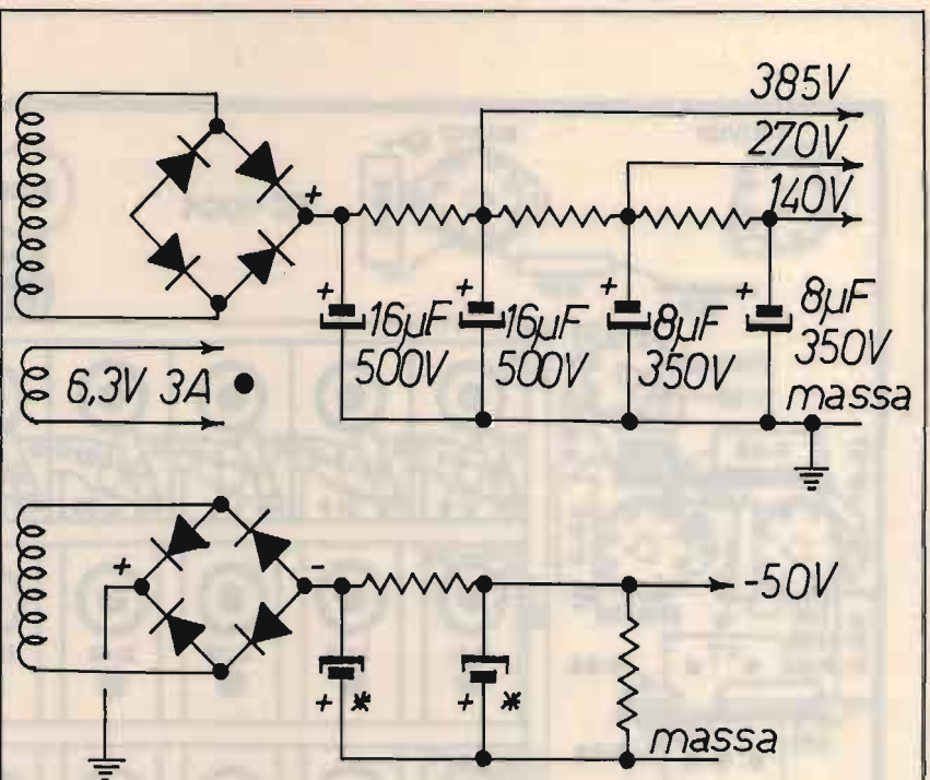
figura 4 Alimentatore da rete (vedi testo). Impiegare un trasformatore da 120\text{ W} circa. ★ = a scelta ● = accensione diretta.
