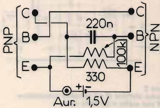
figura 3 Schema elettrico (a sinistra), e prototipo (a destra) di un provatransistori dinamico NPN/PNP.
