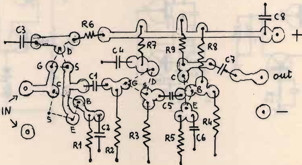
figura 4 Il circuito stampato, visto in trasparenza dal lato componenti. Per maggior chiarezza non è stata disegnata la zona di massa, che circonda lateralmente le piste.
