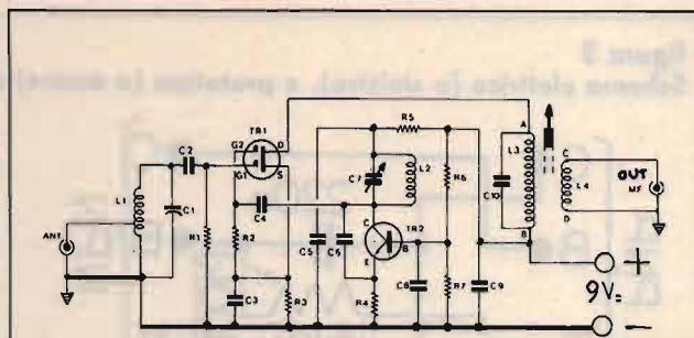
figura 2 Schema elettrico di un semplice convertitore VHF con uscita a 30 MHz circa.
