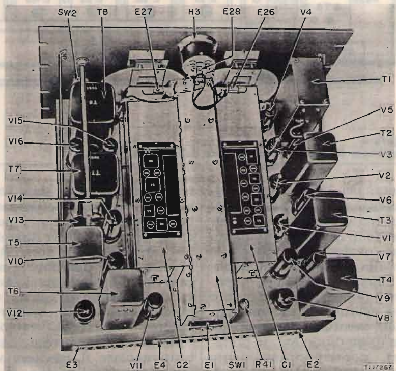
figura 5 Vista dall'alto dello chassis dell'apparecchio BC1004.
