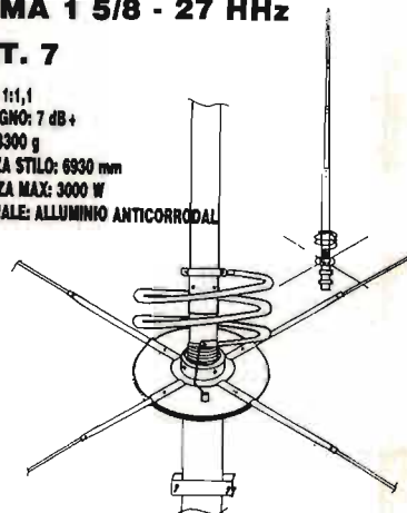
ROMA 1 5/8 - 27 HHz
