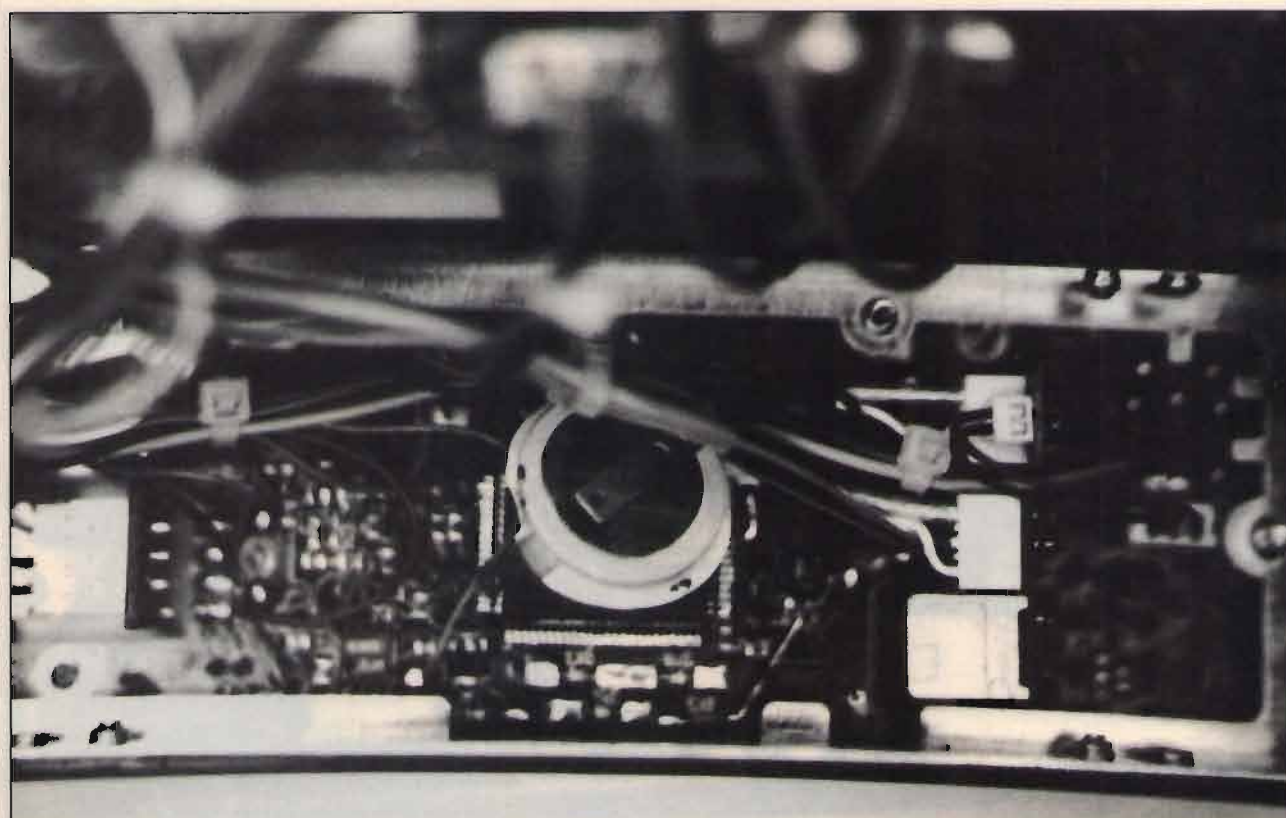
figura 4 Per poter accedere ai diodi da rimuovere, è necessario dissaldare la batteria al litio.
