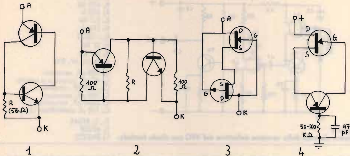
figura 1 Il circuito 1, senza resistenza, rappresenta lo schema di principio, però senza la R non funziona. I transistori usati, per una R di 56 Ω, erano un OC 75 e un AC 127. Il circuito 2 è da preferire, specie quando i transistori usati nel circuito 1 non danno buoni risultati. La R va trovata sperimentalmente, il suo valore varia tra i 50 e i 60 Ω. Il circuito 3 è lo schema di principio per i fet. Il circuito 4 lo sostituisce, comunque, con ottimi risultati.
