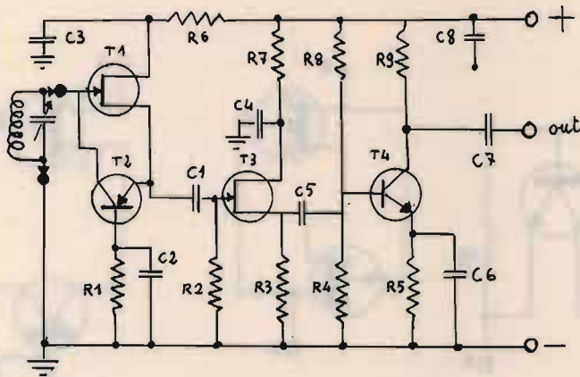
figura 3 Schema elettrico della versione definitiva del VFO con diodo lambda.
