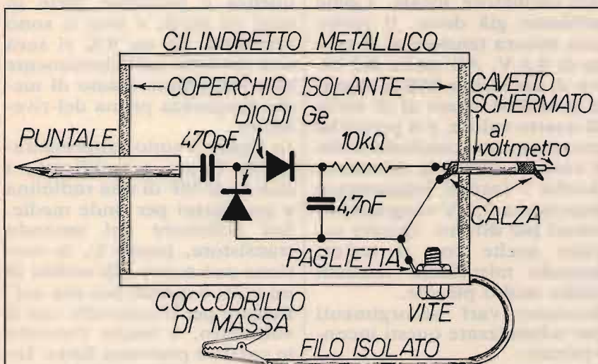
figura 1 Schema e dettagli costruttivi di un probe a radiofrequenza. I due diodi sono al germanio e vanno selezionati per aumentare la sensibilità del probe.
