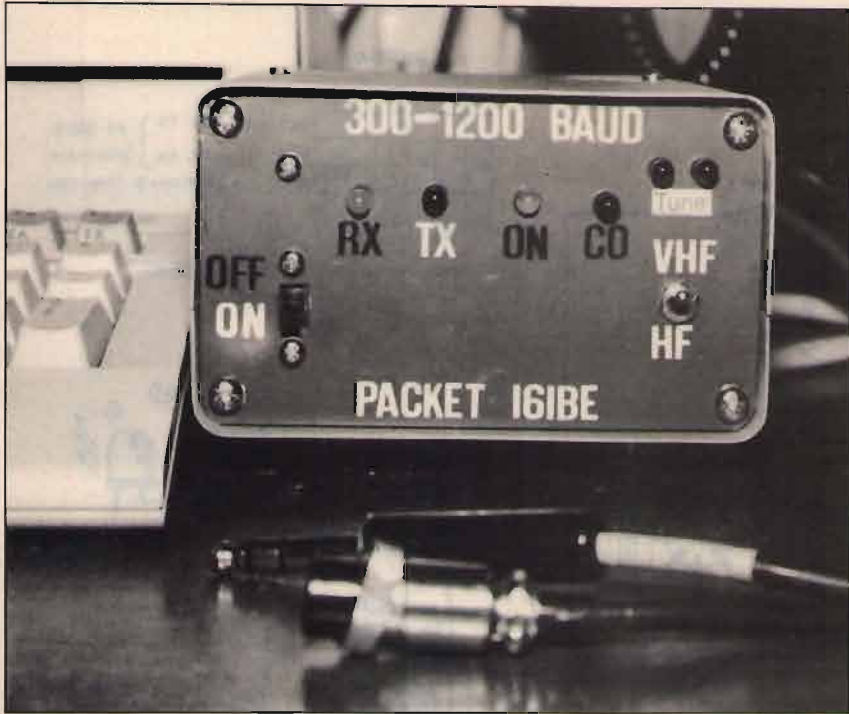
foto 2 Modem finito.
