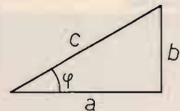
figura 6 Il coseno è il rapporto fra il lato a e il lato c .
