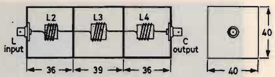
Schema elettrico e realizzazione pratica del filtro Chebyshev.
