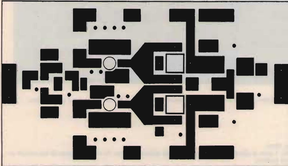
Parte superiore del rame (dove verranno sistemati i componenti) della piastra del circuito stampato per la realizzazione dell'amplificatore.
