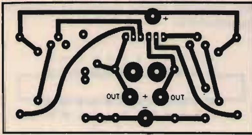
Rame della piastrina del circuito stampato dove si trovano i due circuiti che forniscono le due tensioni di polarizzazione. Dimensioni: 5/6 del naturale.
