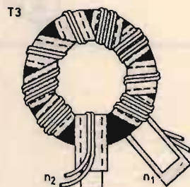
Realizzazione pratica di T_3
