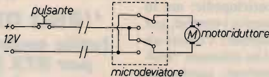
microdeviatore
