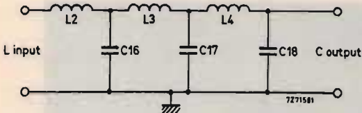
Schema elettrico e realizzazione pratica del filtro Chebyshev.
